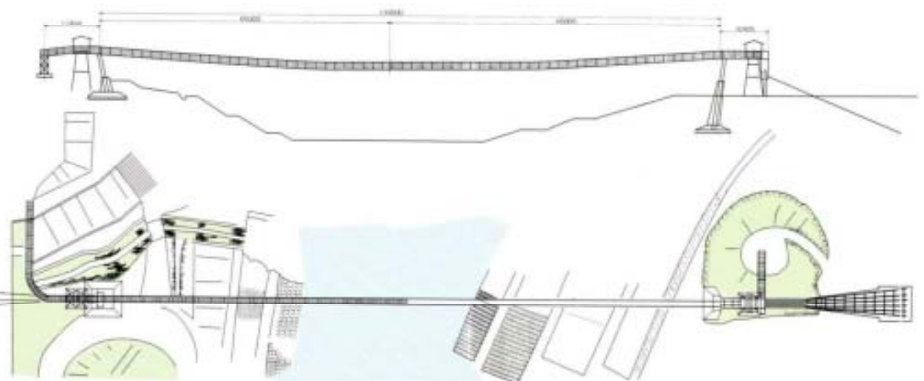
汗の原親水公園吊り橋全体図
