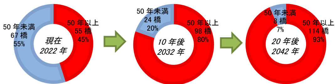
建設後50年以上の橋梁数の増加
