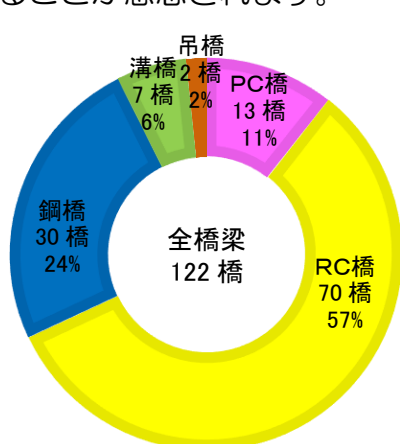
橋種別の橋梁割合
